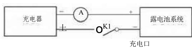
图 4 充电口错接保护试验示意图
