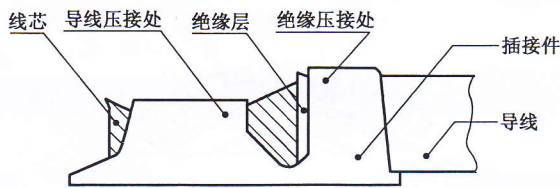
图 1 导线与插接件的压接连接
